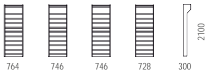
P220 P221 P221 P222 Single Left Right Middle
